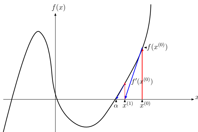
図 1: ニュートン法概略図. x^{(0)} は初期値, x^{(1)} は次の値. 青線は f' の勾配をもちかつ f(x) を通る一次関数であり, 実際の解は \alpha である.
