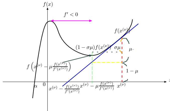
図 2: 減速ニュートン法. ピンクの領域に x^{(\nu+1)} が行かないように f\left(x^{(\nu)} - \mu^{(\nu)} \frac{f(x^{(\nu)})}{f'(x^{(\nu)})}\right) で評価して, f\left(x^{(\nu)} - \mu^{(\nu)} \frac{f(x^{(\nu)})}{f'(x^{(\nu)})}\right) < (1 - \sigma\mu^{(\nu)})f(x^{(\nu)}) という制限を掛けている.
