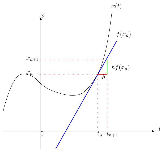
図 1: オイラー法概念図. 青線は点 (t_n, x_n) での傾き f(x_n) の直線. t_{n+1} のときの値 x_{n+1} が x(t_{n+1}) での値と同じと近似して計算していく.
