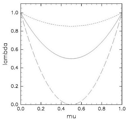
図 3: (25) 式に関する波長と増幅係数の関係. 縦軸は |\lambda|^2 , 横軸は \mu である. 破線は L = 2\Delta x , 実線は L = 4\Delta x , 点線は L = 8\Delta x の場合である.
