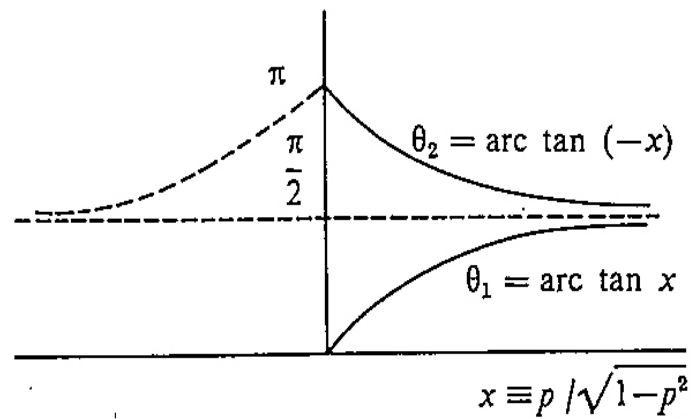
図 1: リーフログスキームにおける物理モードと計算モードの位相の振る舞い (Mesinger and Arakawa (1976) より引用). 縦軸は位相, 横軸は x = p/\sqrt{1-p^2} である.
