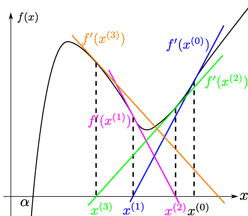
図2 ニュートン法が収束しない例. \alpha が求めたい解. x^{(0)} から始めて, 解を求めようとする, 途中で勾配 f' が負になってしまい, 収束しない.
