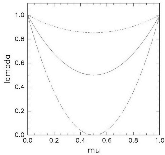
図 3: (55) 式に関する波長と増幅係数の関係. 縦軸は |\lambda|^2 , 横軸は \mu である. 破線は L = 2\Delta x , 実線は L = 4\Delta x , 点線は L = 8\Delta x の場合である.
