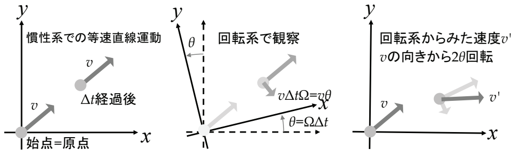
図 4.2 コリオリ力の考え方. 慣性系の等速直線運動 (左) は回転系から観察すると加速度を持つ (中, 右). この加速度がコリオリ力である. この例では簡単のため, 質点の初期位置は回転軸を通る原点に一致させている.
