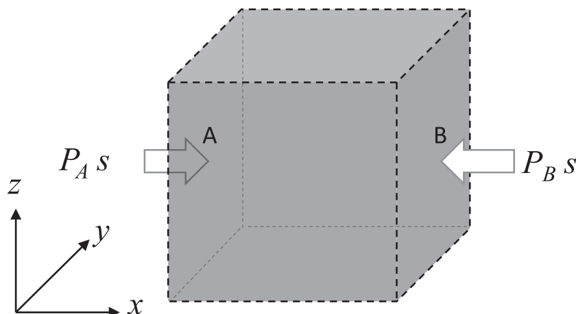
図4.1 気圧傾度力の考え方。もし P_A > P_B なら、微小立方体には右向きに合力が働く。これが気圧傾度力である。
